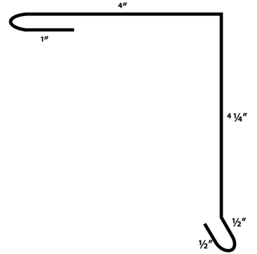
Z-Bar Rake
