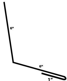
Endwall
